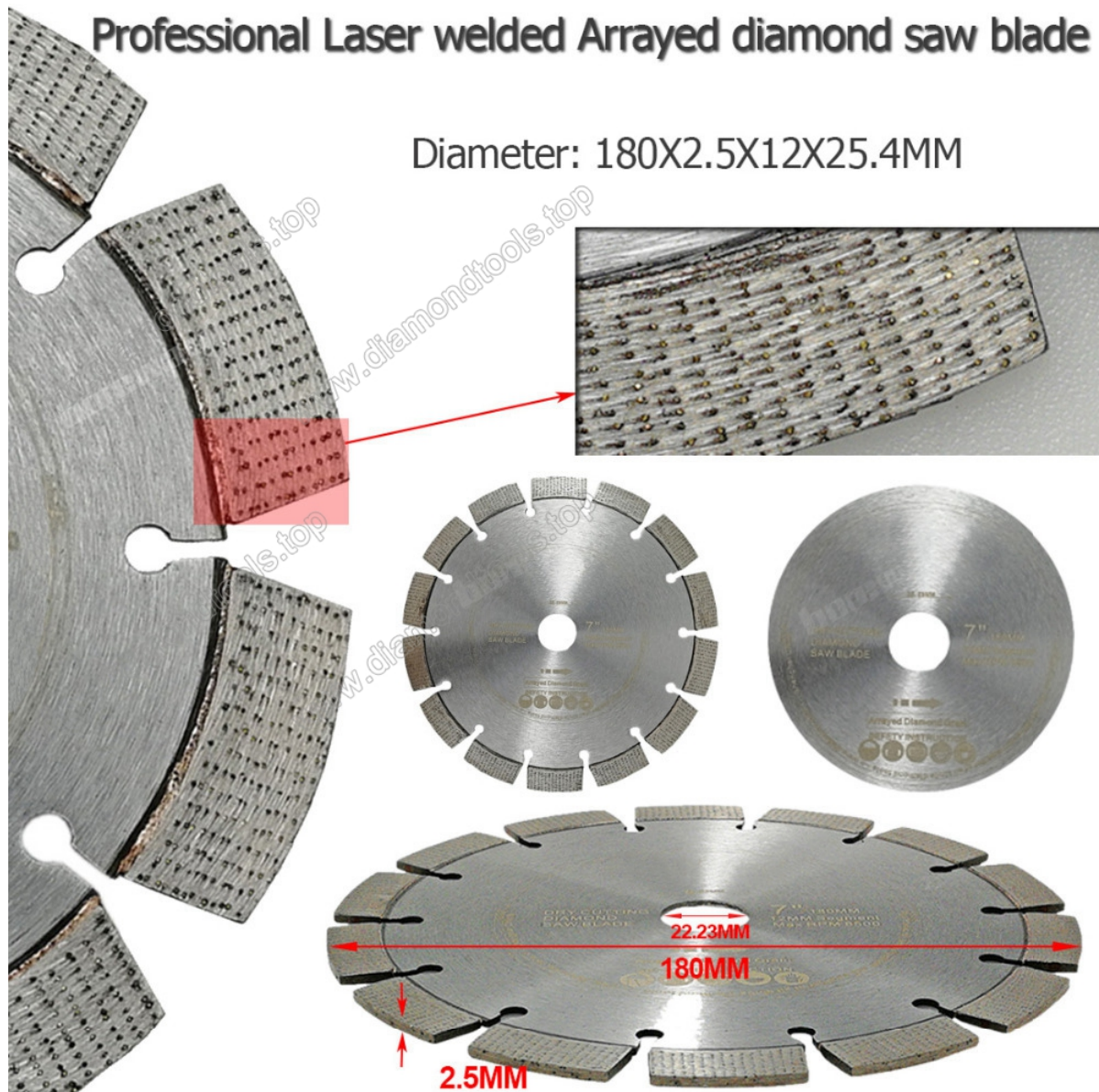
9inch Лазерная сварка алмазного пильного диска
