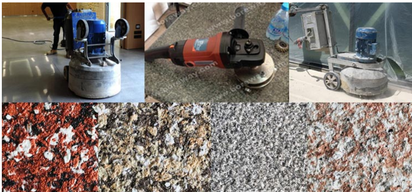
Алмазный абразивный инструмент Буш Молотковый валик
