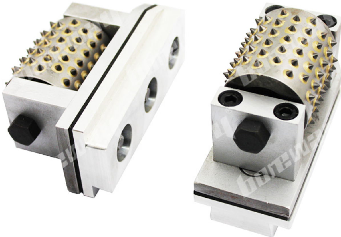
Rollenkopf mit 99 Segment Zum Schleifen und Kalibrieren der Steinplatten wie Granit, Marmor usw.
