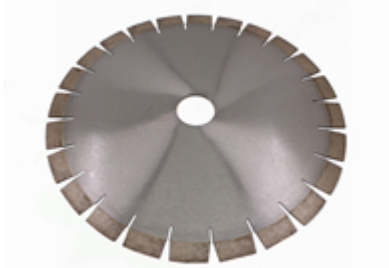
D350 * 3.2 * 20 * 40 mm * 50/60 mm Schrägschneidsäge
